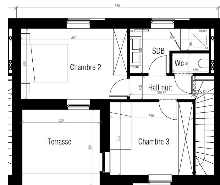
ÉTAGE
