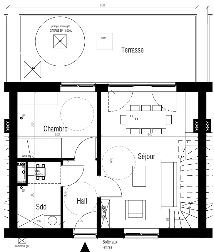
REZ-DE-CHAUSSÉE
