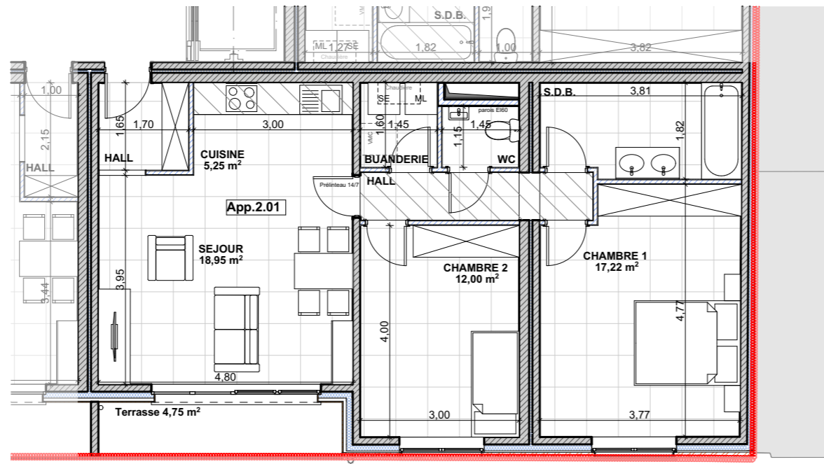
Plan appartement
