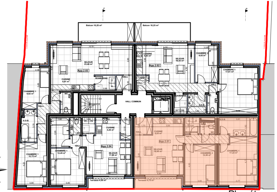
Plan étage
