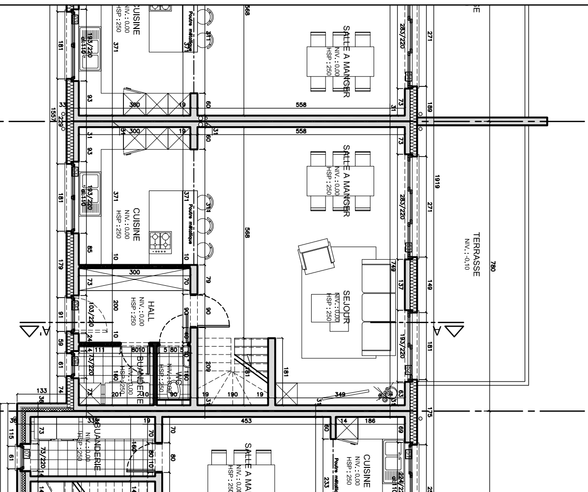
PE I LOGEMENT 2 - TYPE I
