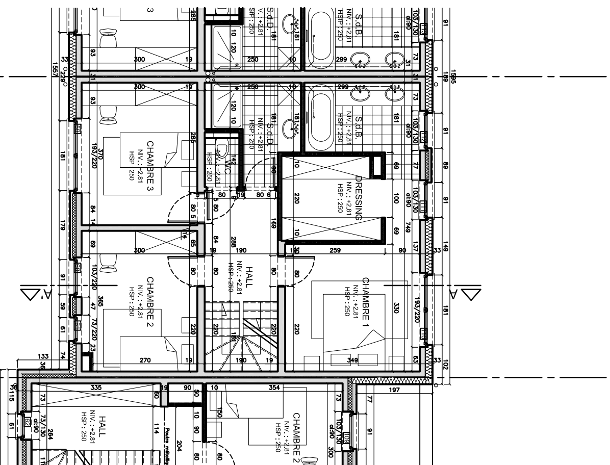
LOGEMENT 2 - TYPE I
