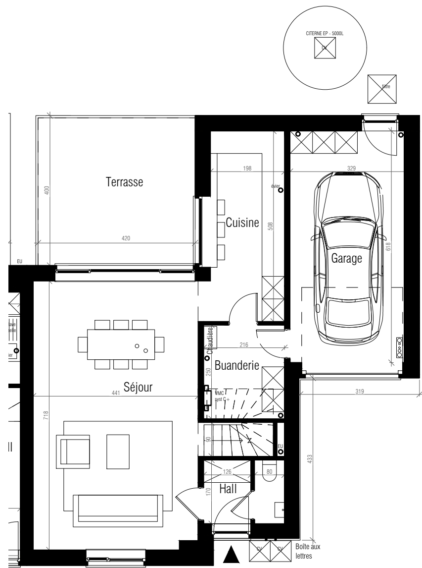
REZ-DE-CHAUSSÉE
