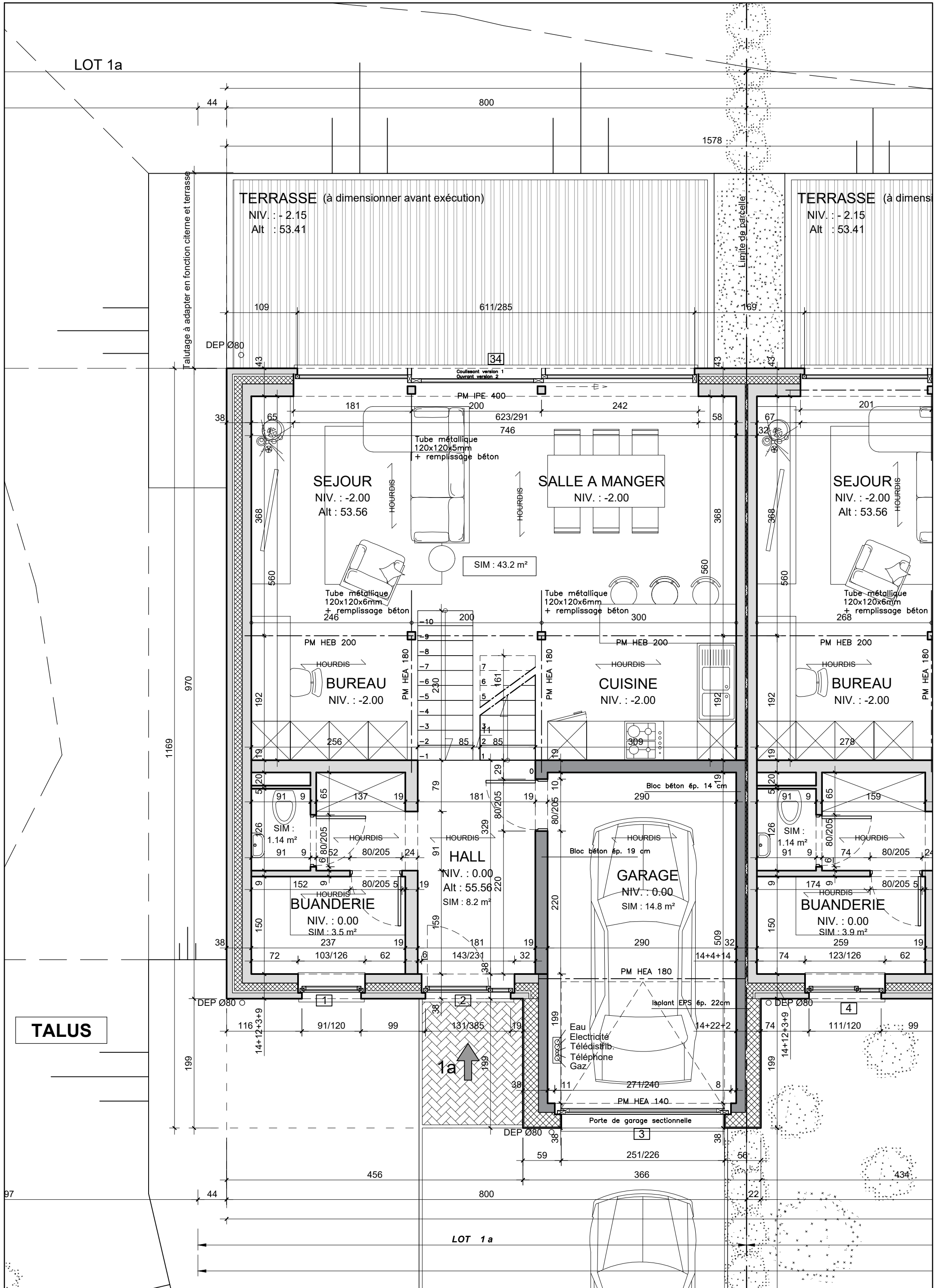
Plan Lot 1a - Rez-de-chaussée - Echelle 1/50 Situation projetée
