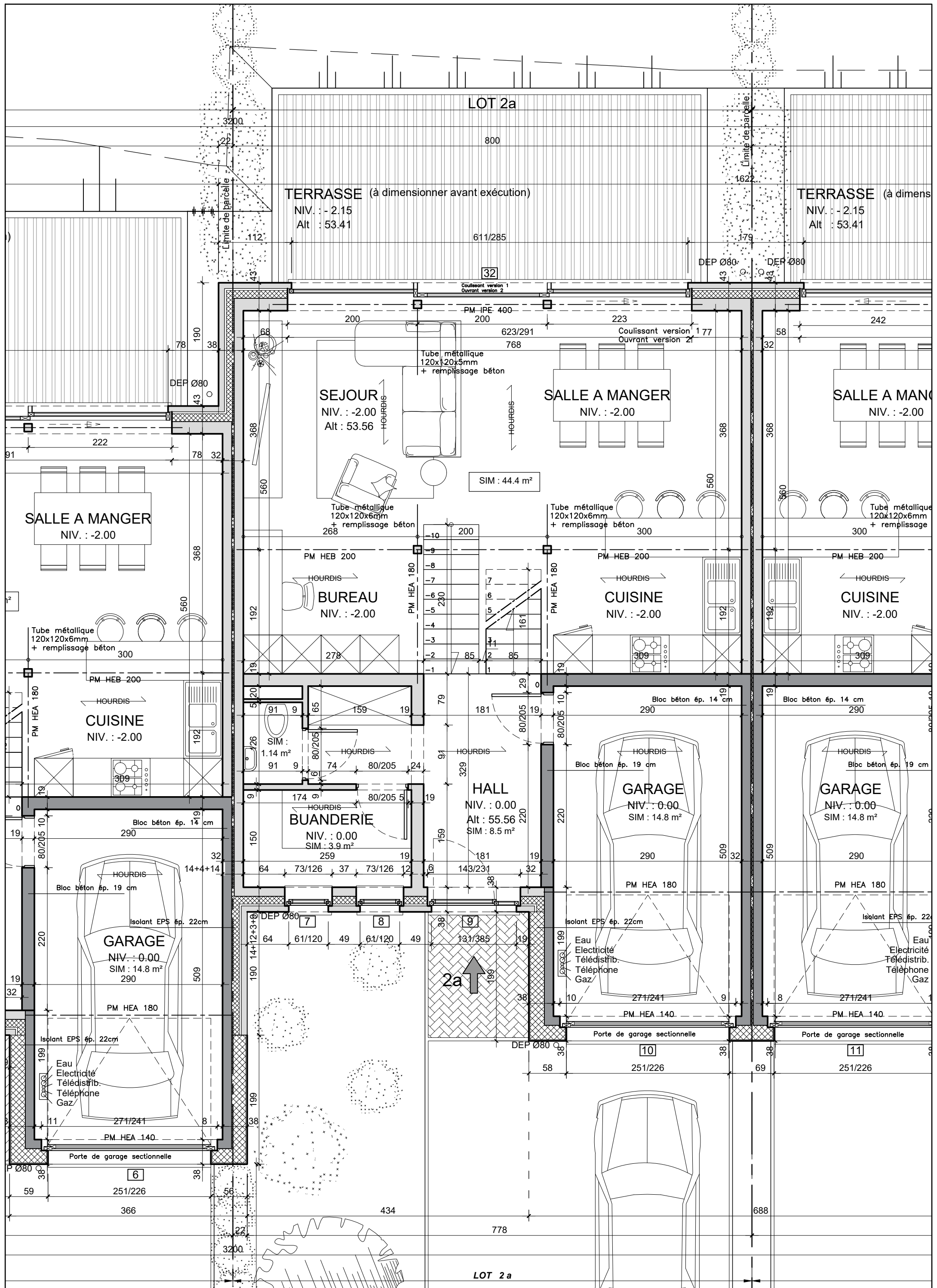
Plan Lot 2a - Rez-de-chaussée - Echelle 1/50 Situation projetée
