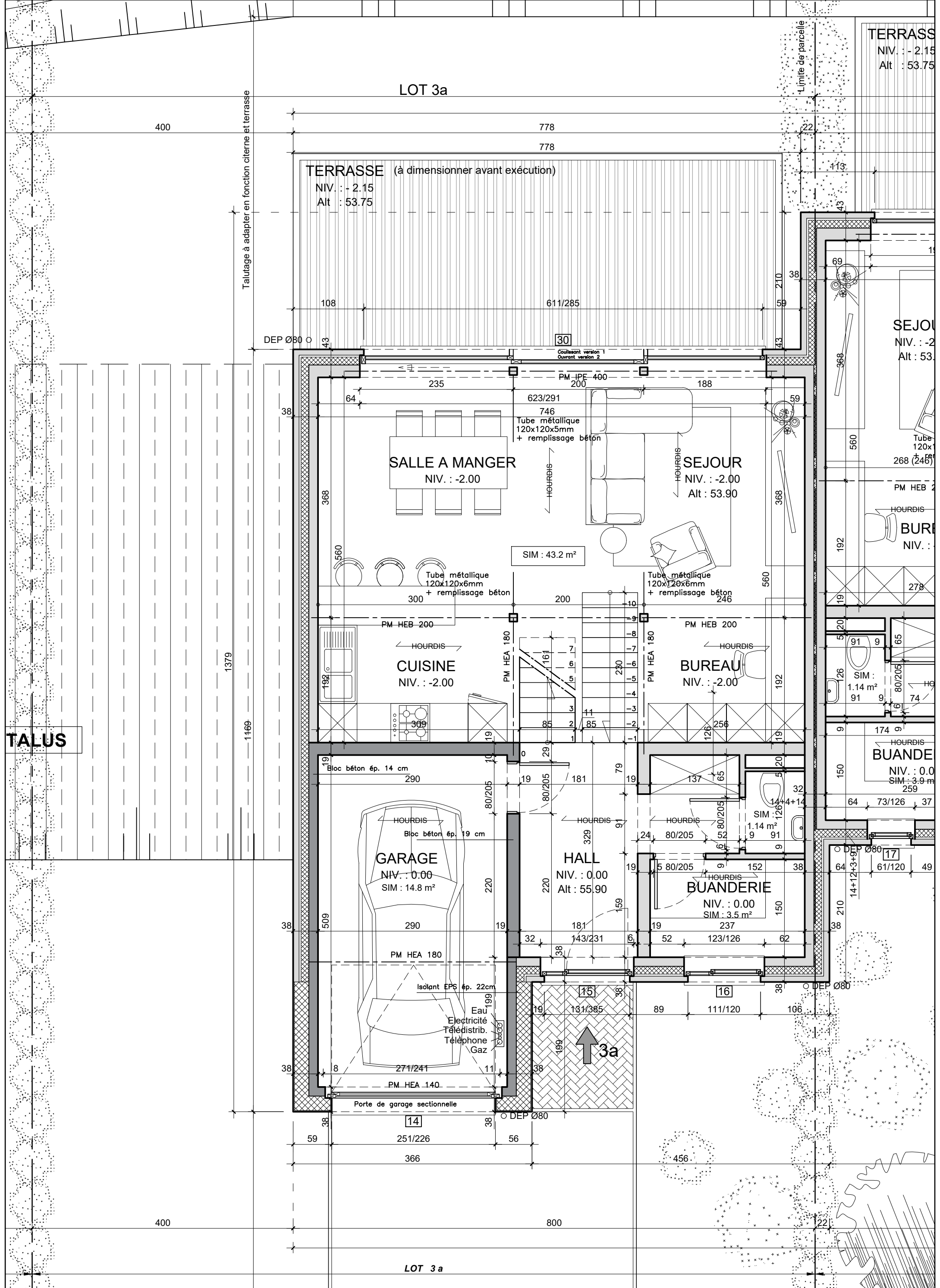
Plan Lot 3a - Rez-de-chaussée - Echelle 1/50 Situation projetée
